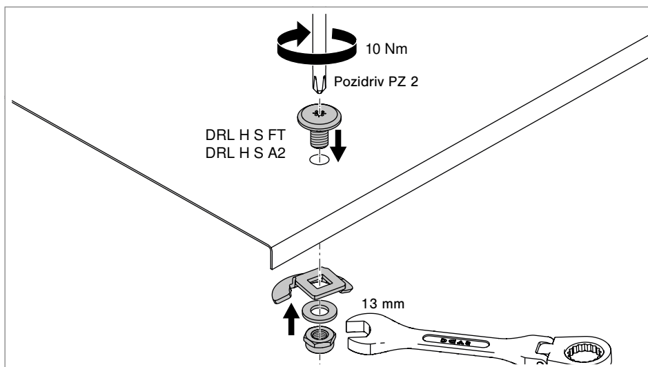
Slika 87: Učvršćivanje obrtne brave zavrtanjima
