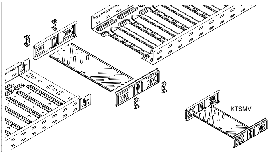
Slika 21: Brza spojica KTSM
