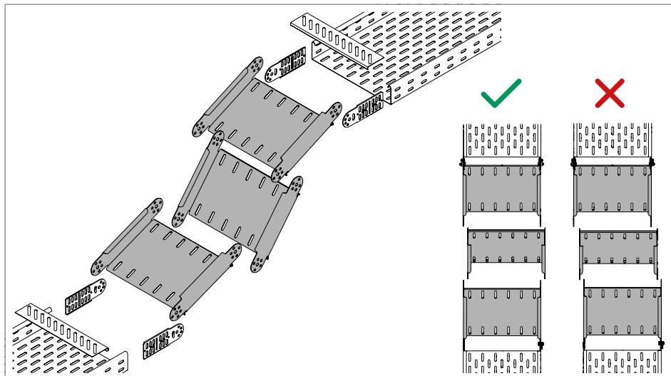
Slika 69: Element zglobne krivine sa polovinom zglobne spojnice i podnim završnim limom
