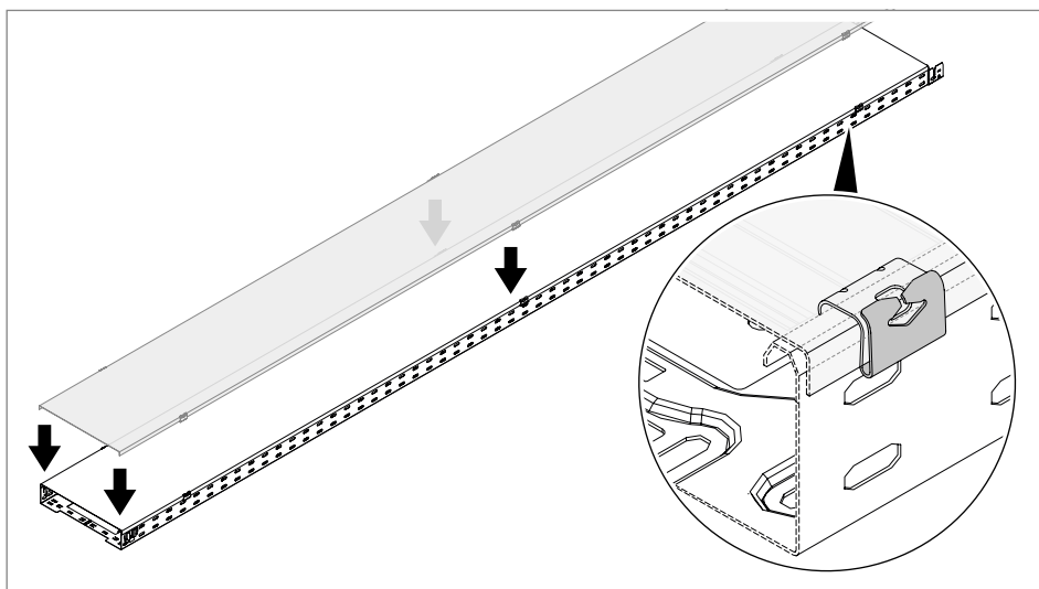
Slika 85: Uglavljivanje poklopca na mesto
