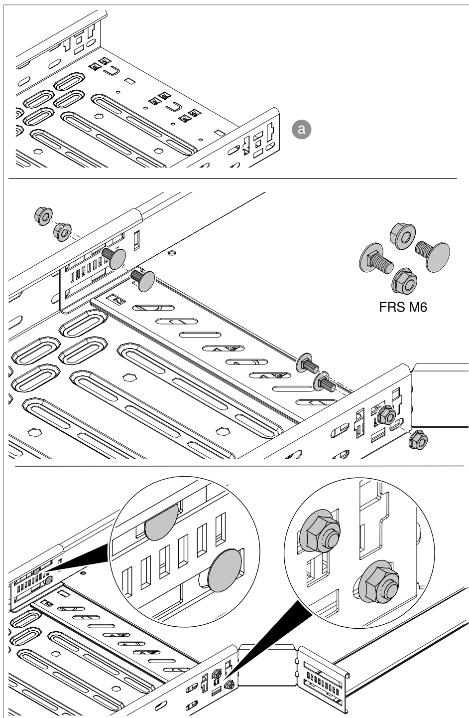
Slika 48: Učvršćivanje faznskog komada zavrtnjima (nerezani nosač kablova (a))
