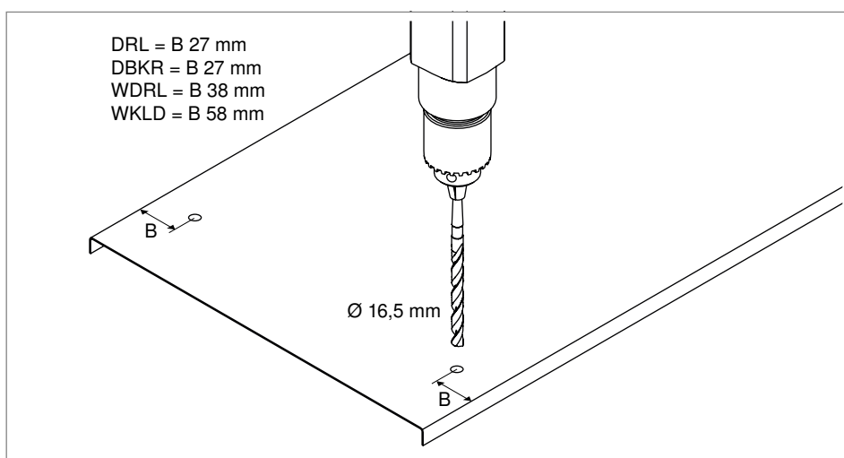
Slika 86: Prethodno bušenje poklopca
