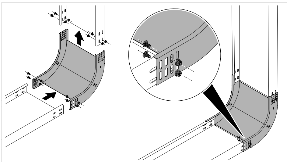
Slika 68: Montaža vertikalne krivine sa uzlaznim nagibom
