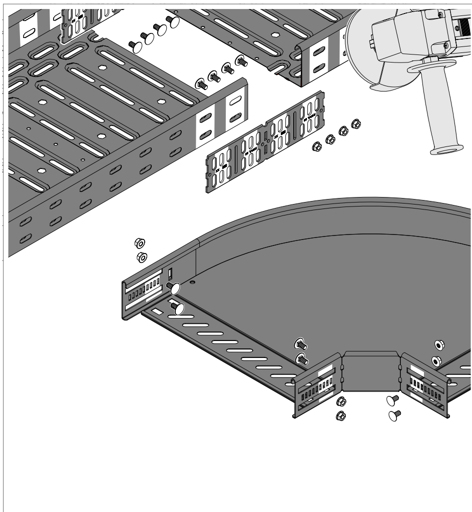
Slika 18: Ukloniti plastifikaciju
