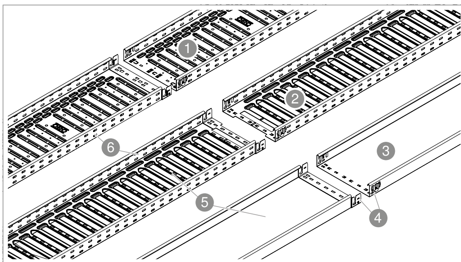
Slika 1: Perforirani i neperforirani nosači kablova
