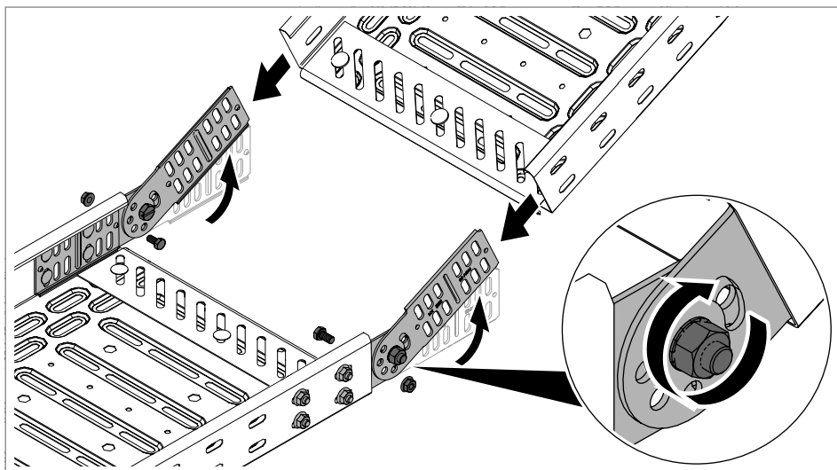
Slika 41: Zategnuti zglobni zavrtnanj
