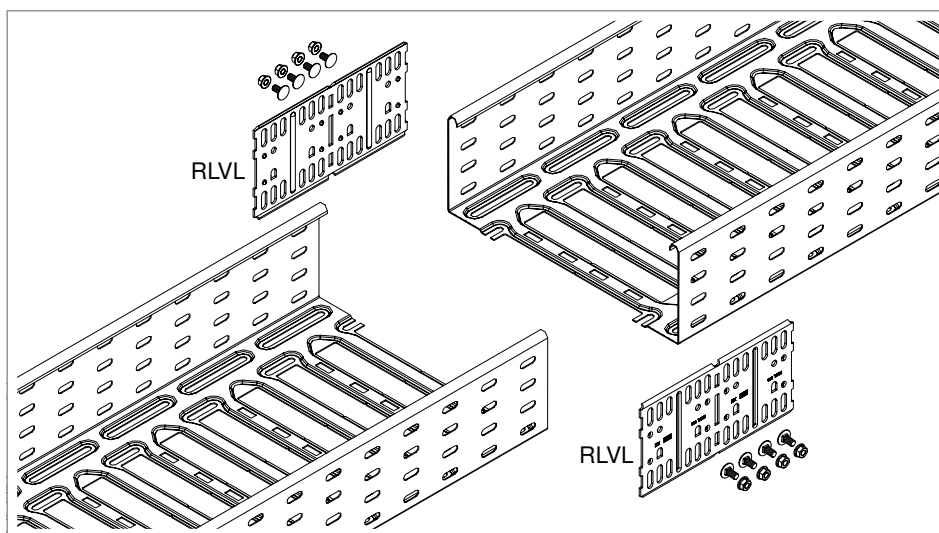
Slika 27: Brza spojica RLVL
