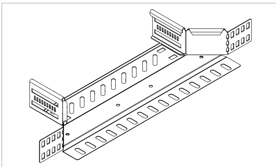
Slika 5: Ugradna račva
