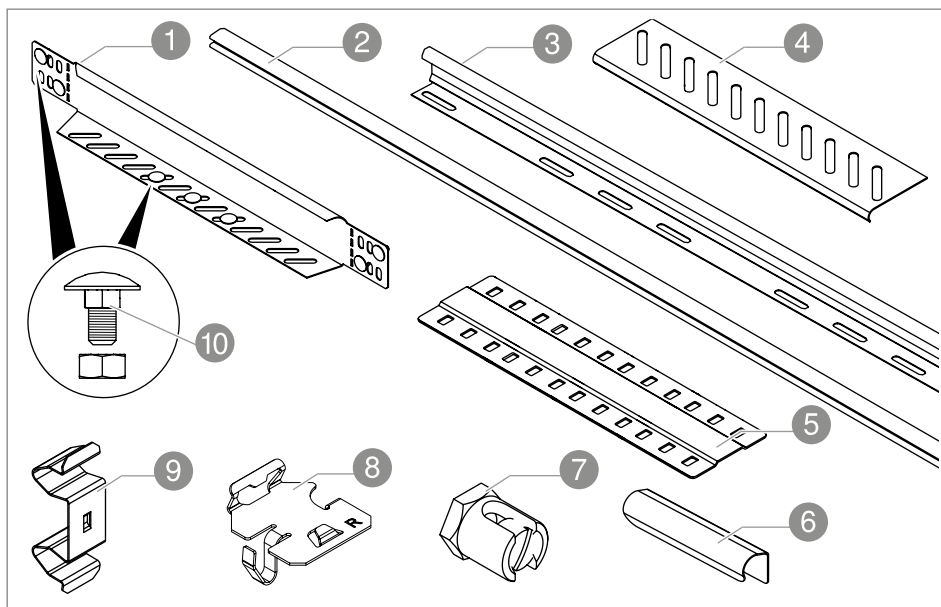
Slika 15: Pribor
