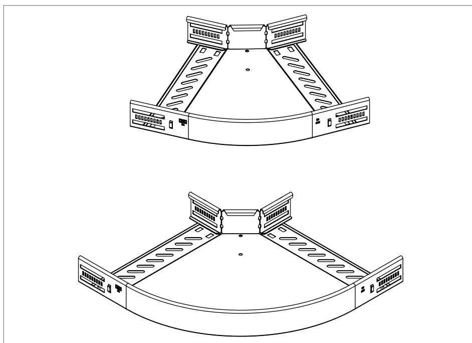
Slika 3: Krivina 45° i 90°
