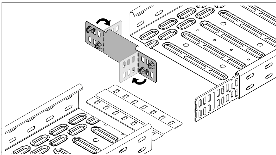
Slika 73: Savijanje reducira
