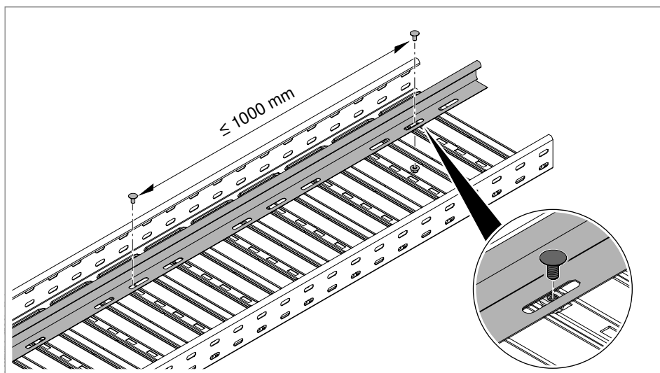
Slika 78: Učvršćivanje pregrade zavrtnjima
